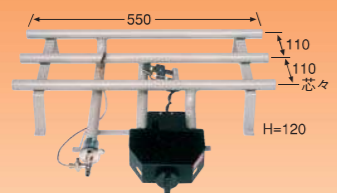
カウンター用3本バーナー 半自動
